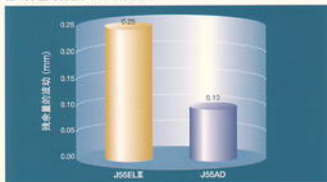
■ 注塑产品重量的偏差 (本公司内比较)
