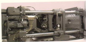
锁模装置
